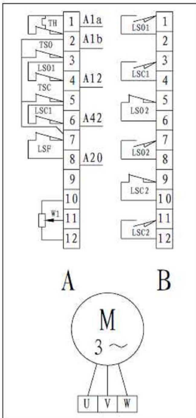
Рис. 15 Схема монтажа кабеля для электропривода взрывозащищенного исполнения
