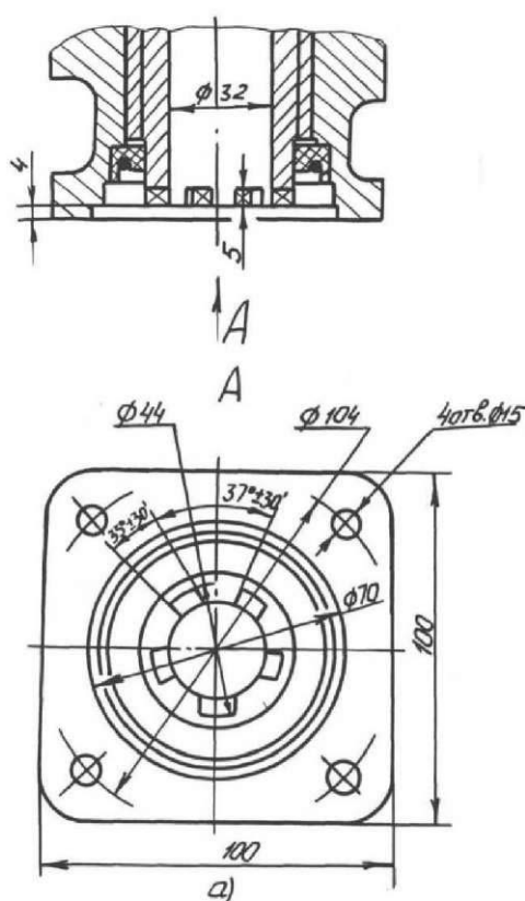
Присоединительные размеры фланца электропривода МЭП типа А
