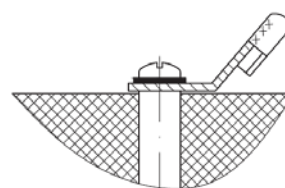
Рис. 15 Схема монтажа кабеля для электропривода взрывозащищенного исполнения
