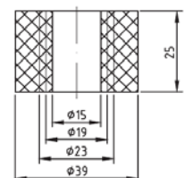
Рис.16 Уплотнительное кольцо
